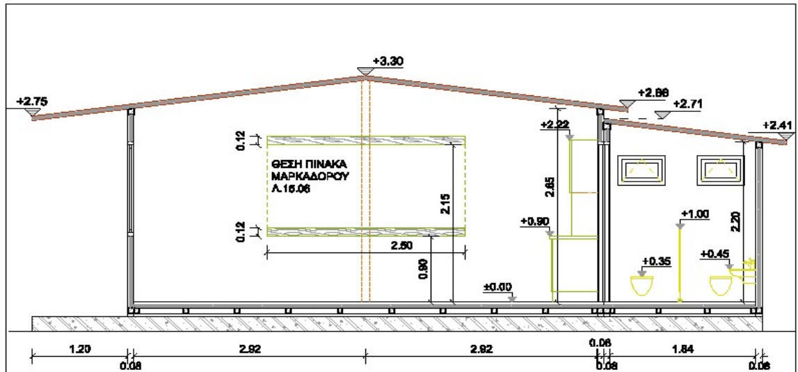
ΤΟΜΗ Τ1-Τ1
