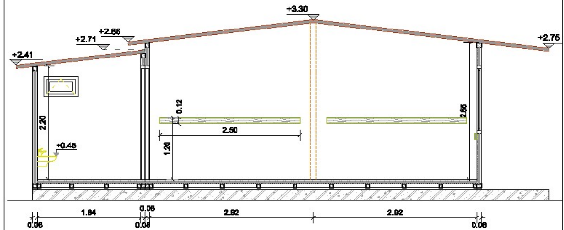
ΤΟΜΗ Τ2-Τ2
