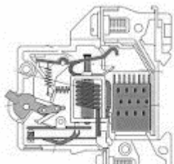
Εικόνα 16 Μικροαυτόματος 25 Α ράγας
