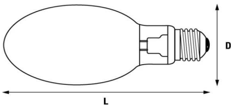
Εικόνα 1 250W SOD D=91mm L=227mm
