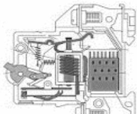
Εικόνα 14 Μικροαυτόματος 16 Α ράγας
