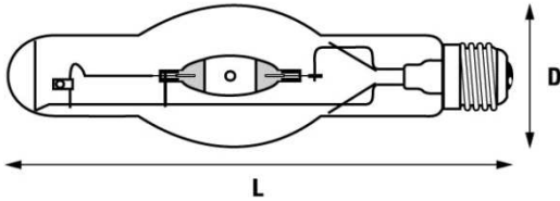
Εικόνα 2 4000w HQI D=63mm L=270mm
