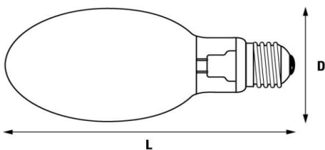
Εικόνα 2a 250W Hg D=91mm L=228mm
