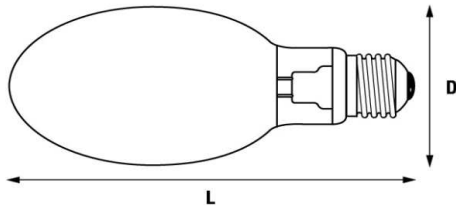
Εικόνα α23 500W Hg D=122mm L=275mm
