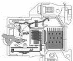
Εικόνα 15 Μικροαυτόματος 20 Α ράγας
